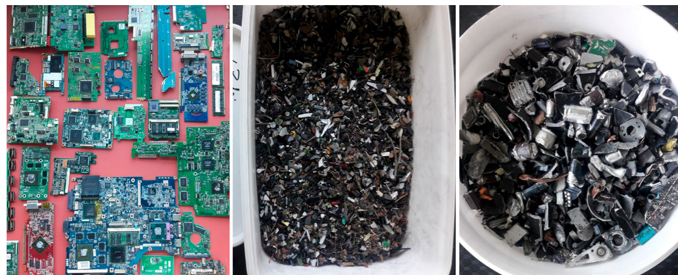
Figure 4: exemples de fractions générées (de gauche à droite): circuits imprimés de la classe 1, après le démontage fin, obtenus à partir d'appareils électroniques modernes; fractions de matières plastiques extraites dans l'essai par lots avec une forte teneur en métaux précieux (importante proportion de circuits imprimés); fraction d'aluminium obtenue dans l'essai par lots avec un séparateur à courants de Foucault. On peut distinguer de nombreux condensateurs électrolytiques qui ont, certes, été un peu abîmés à l'ouverture, mais qui ont été pratiquement tous séparés dans cette fraction.
